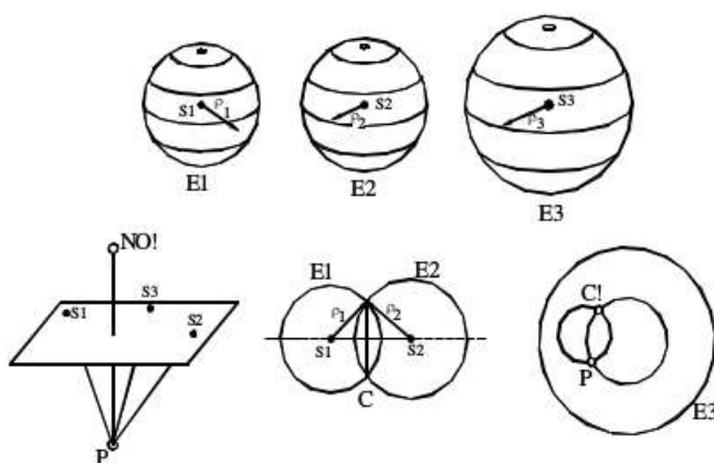
Figura 2.2: Las letras S indican la posición de los satélites, las \rho las distancias entre satélite-receptor, y la letra P la del punto cuyas coordenadas se quiere conocer, es decir la ubicación del receptor GPS. Fuente:[4]
