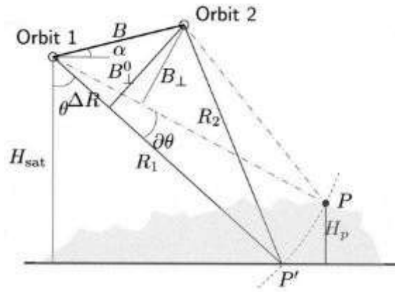
Figura 2.9: Configuración interferométrica. Fuente [7]
