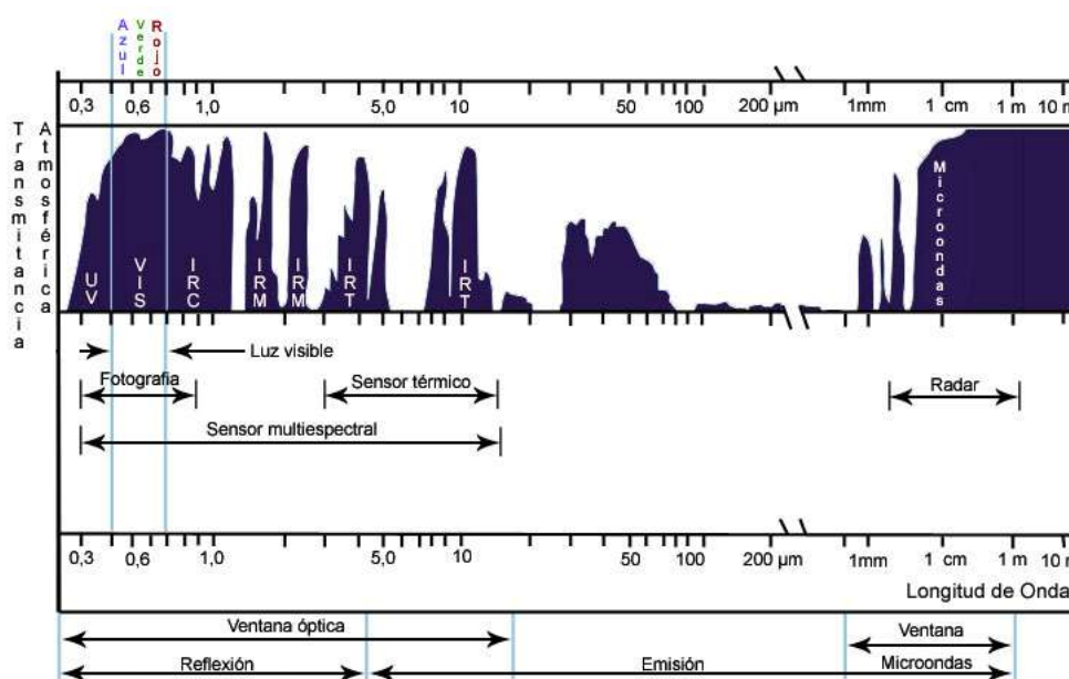
Figura 2.7: Ventanas atmosféricas del espectro electromagnético
