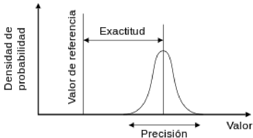
Figura 2.1: Valor de referencia, densidad de probabilidad, exactitud y precisión. Fuente:Wikipedia
