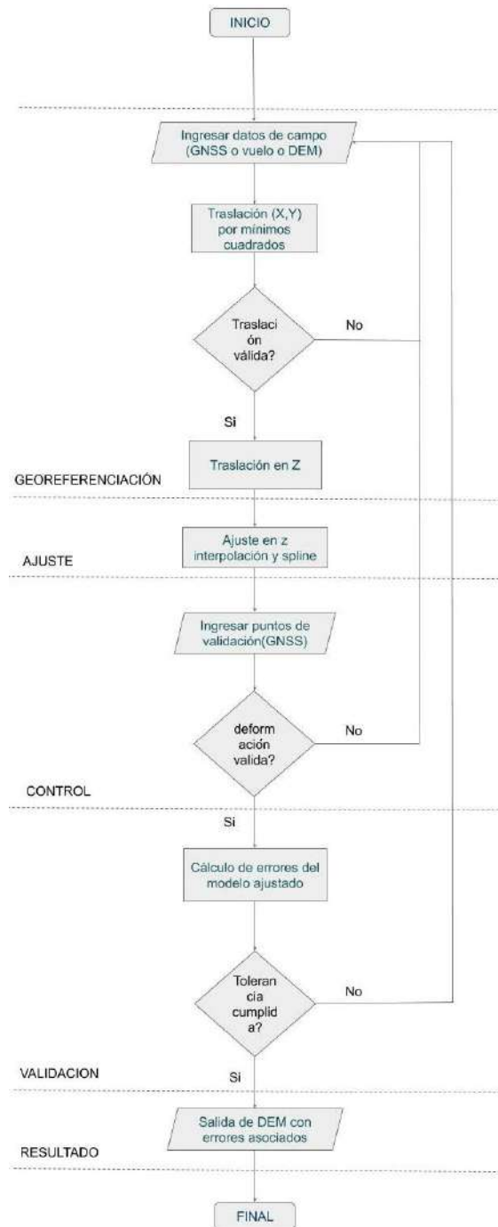
Figura 4.8: Algoritmo de trabajo desarrollado. Fuente: Elaboración propia
