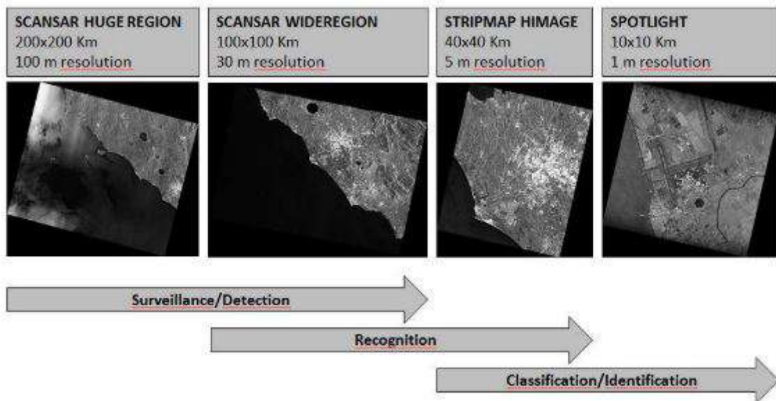
Figura 2.11: Modos de adquisición de los sensores COSMO-SkyMed. Fuente: [9] página 8
