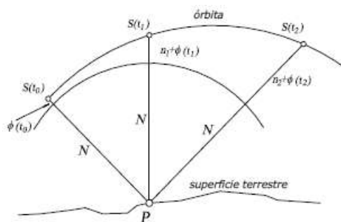
Figura 2.3: Ciclos enteros y decimales de fase en cada instante t_n con P el punto donde se ubica el receptor. Fuente:[4]
