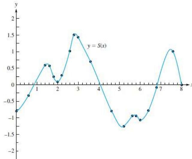
Figura 2.18: Spline cúbico. Fuente:[12]
