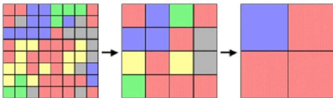
Figura 2.13: Remuestreo de distancia interpíxel. Fuente: internet
