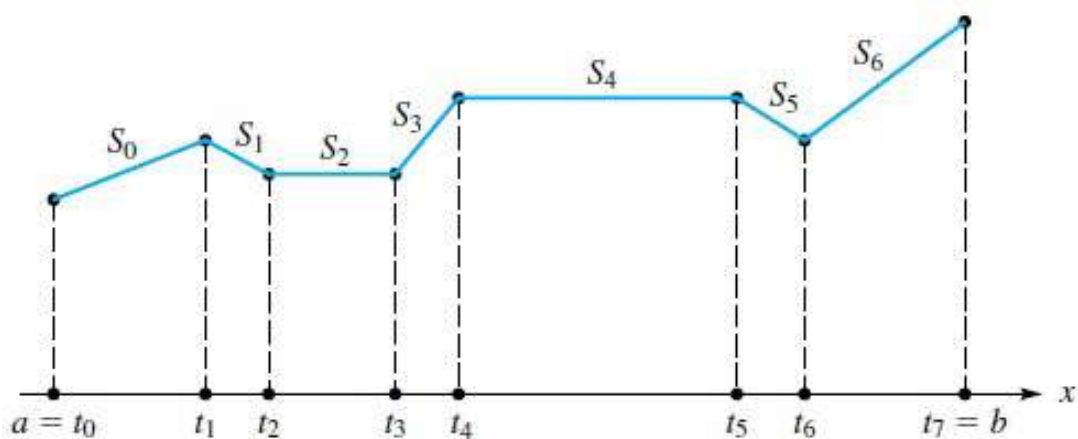
Figura 2.15: Interpolación lineal por partes. Fuente: [12]
