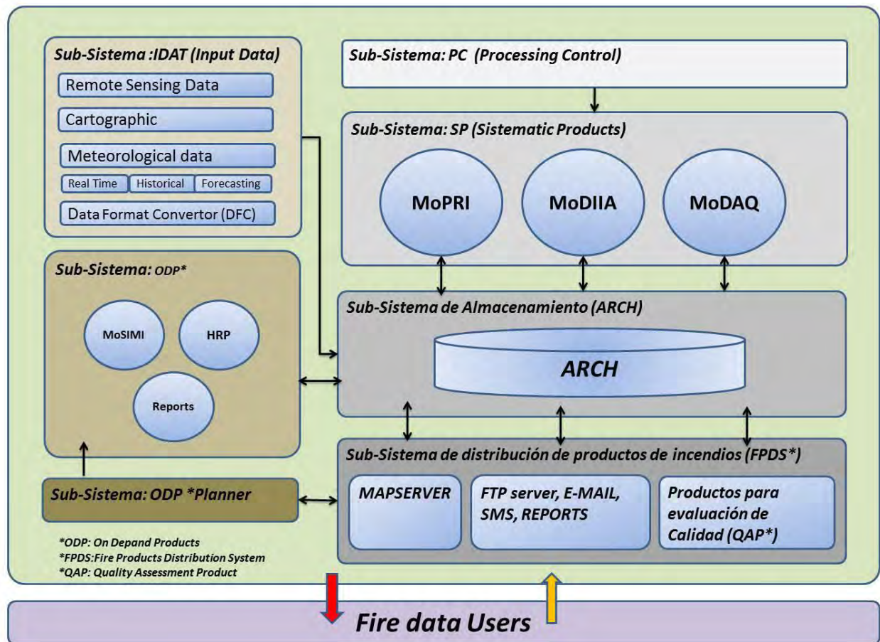
Figura 9: Arquitectura del Sistema SARTiv.
