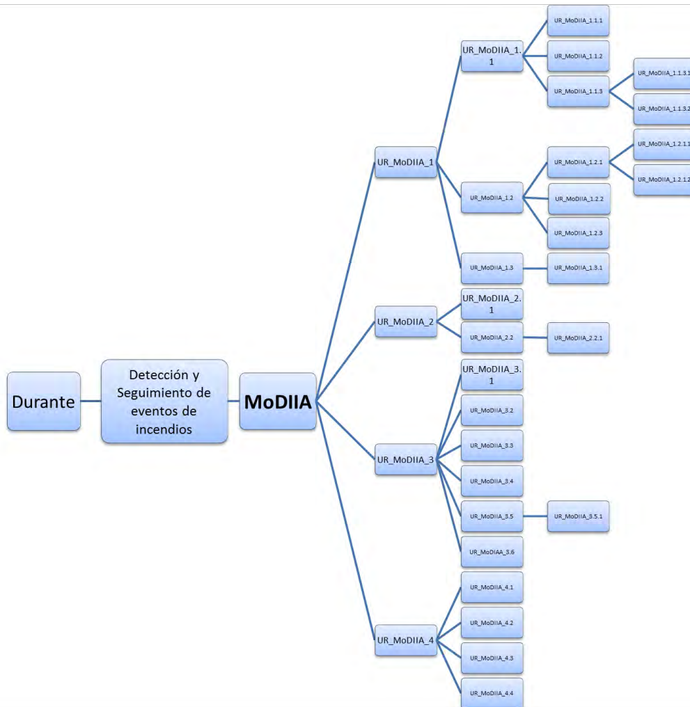
Figura 5: Esquema de la estructura sobre los requerimientos de usuarios correspondiente al módulo MoDIIA.
