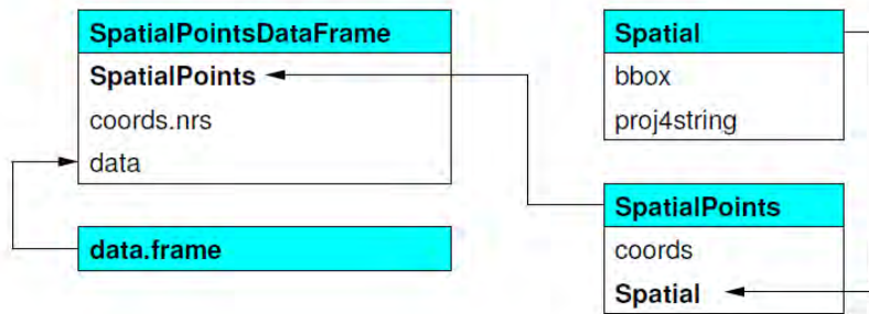
Figura 10: Clases espaciales de Puntos, y sus componentes (slots).
