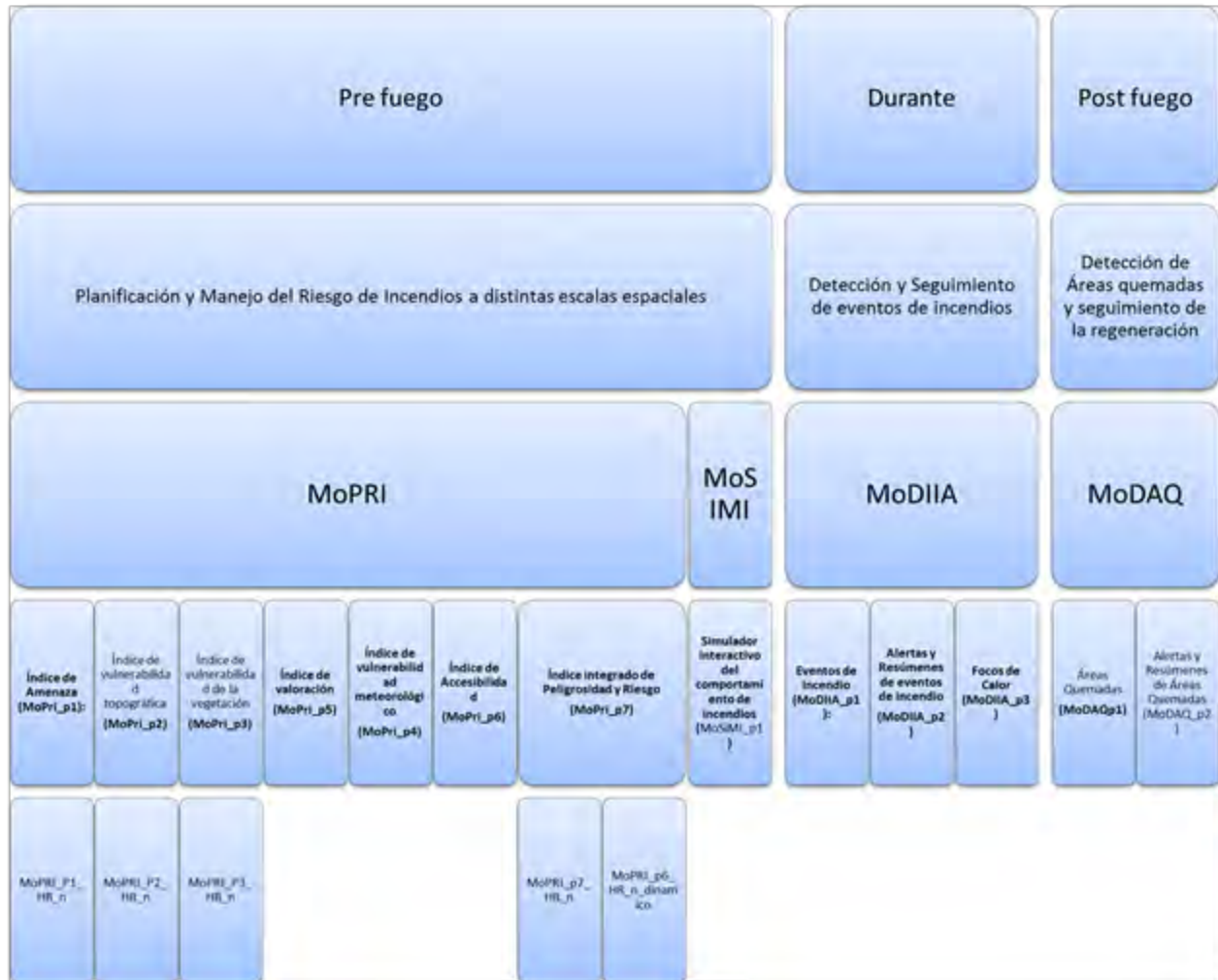
Figura 3: Esquema principal de la organización de los requerimientos de usuarios y productos definidos.
