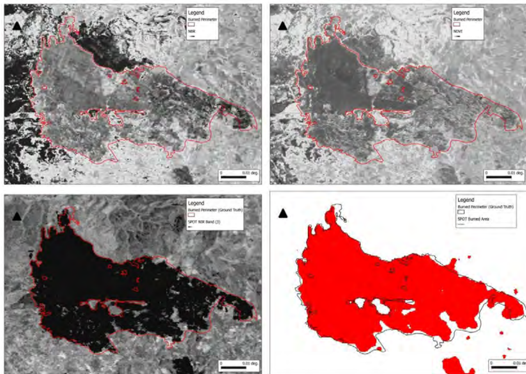
Figura 50: Datos ópticos de SPOT-4; Arriba a la izquierda; Normalized Burned Ratio (NBR). Arriba a la derecha; Normalized Difference Vegetation Index (NDVI). Abajo a la izquierda; Infrarrojo Cercano (IRC). Abajo a la derecha; estimación del área quemada a partir de umbrales de los índices y datos espectrales del IRC.
