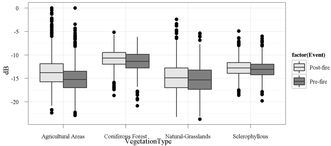
Figura 51: Interacciones entre datos SAR previos y posteriores al incendio con modo de polarización cruzada HH.
