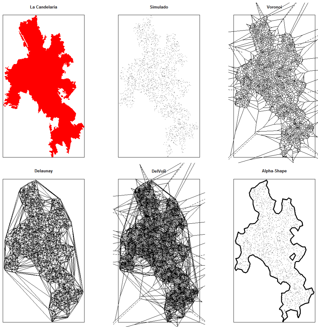
Figura 26: Incendio de La Candelaria, 2003. Los tres paneles de arriba indican de izquierda a derecha la superficie conocida, en el centro la simulación y luego el diagrama de Voronoi. Abajo en el mismo orden se presenta la triangulación de Delaunay, la combinación Delunay-Voronoi, y el resultado del estimador de formas \alpha shape.
