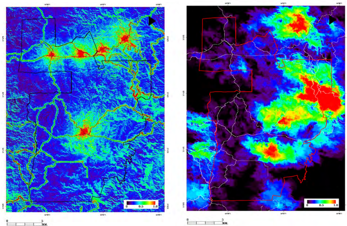
Figura 43: Estimaciones de riesgo de acuerdo a distintos metodos. A la izquierda el índice de riesgo convencional, y a su derecha el índice de peligro de propagación.
