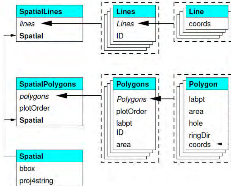
Figura 11: Clases espaciales de Líneas y Polígonos, junto a sus respectivos componentes (slots).
