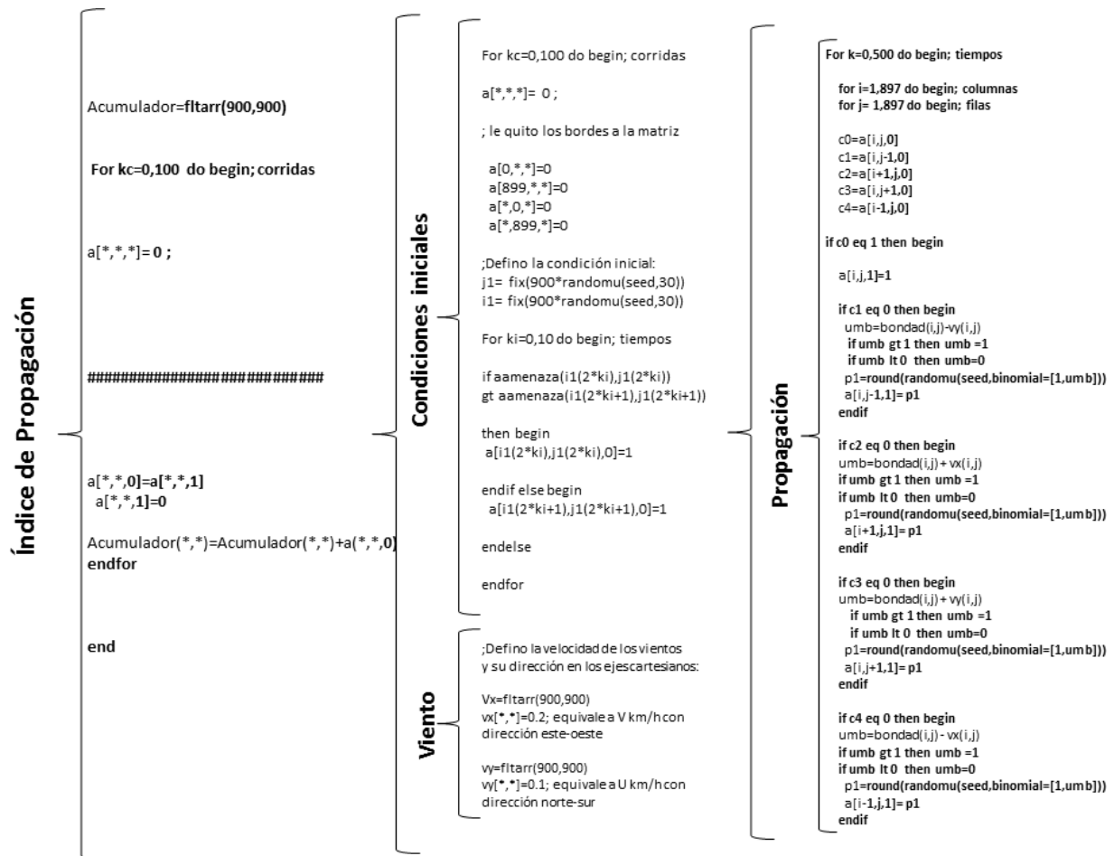
Figura 41: Pseudo código de la aplicación implementada en IDL.
