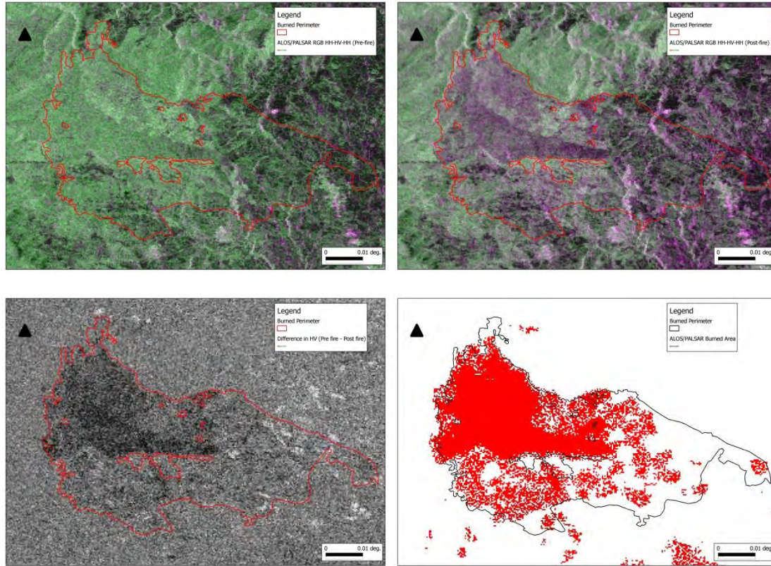
Figura 49: Datos ALOS/PALSAR: Arriba a la izquierda; imagen previa al incendio. Arriba a la derecha; imagen posterior al incendio. Abajo a la izquierda; Diferencia en la polarización HV. Abajo a la derecha; estimación de área quemada por valores de umbrales positivos proveídos por datos de \Delta HV SAR.
