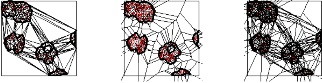
Figura 22: Se presentan simulaciones ppa, donde se ejemplifica el poder de caracterización de la forma del \alpha -shape, presentándose de izquierda a derecha la Triangulación de Delaunay, los diagramas de Voronoi y su superposición.
