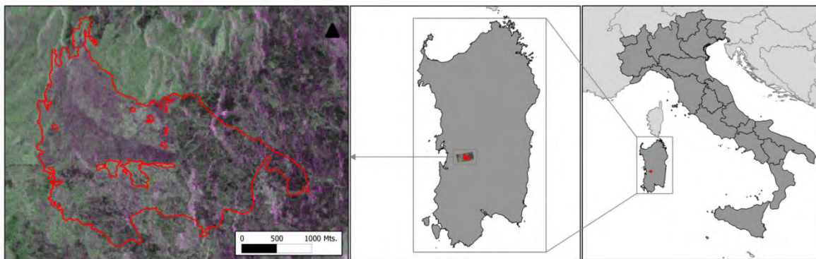
Figura 48: La isla de Cerdeña y el área de estudio con el detalle del perímetro quemado: Imagen ALOS en RGB: HH, HV, HH.
