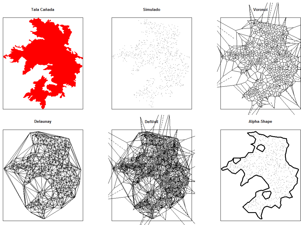
Figura 27: Incendio Tala Cañada, 2003. Los tres paneles de arriba indican de izquierda a derecha la superficie conocida, en el centro la simulación y luego el diagrama de Voronoi. Abajo en el mismo orden se presenta la triangulación de Delaunay, la combinación De Delunay-Voronoi, y el resultado del estimador de formas \alpha shape.
