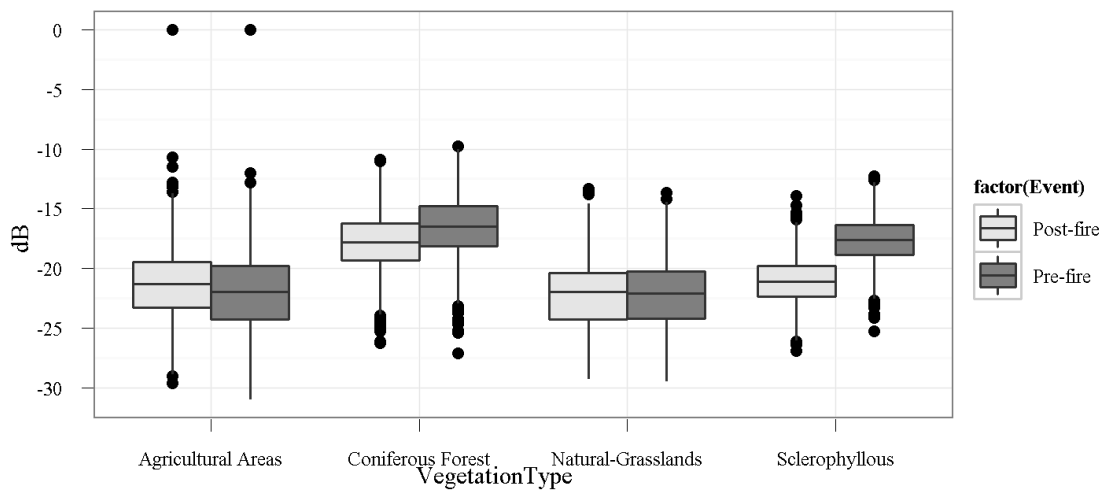
Figura 52: Interacciones entre datos SAR previos y posteriores al incendio con modo de polarización HV.
