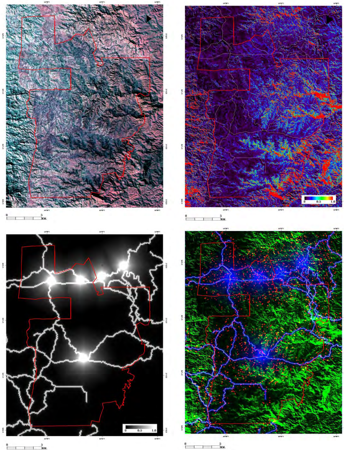
Figura 42: Cartografías sobre las condiciones iniciales planteadas para la simulación de la propagación de incendios. Arriba a la izq. Se presenta la imagen SPOT empleada de base. Arriba a la derecha se presentan los pseudo combustibles. Abajo a la izq. Se presenta la cartografía de amenaza y a la derecha los puntos de ignición.
