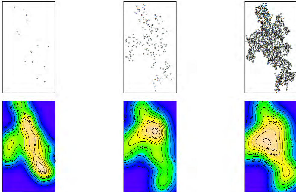
Figura 24: Focos de calor simulados correspondiente al incendio de La Candelaria: Arriba de izquierda a derecha se presentan los resultados de controlar la intensidad \lambda , ajustada a la forma del perímetro conocido. Abajo, en el mismo orden, se representa la estimación de densidad para cada nivel de intensidad.
