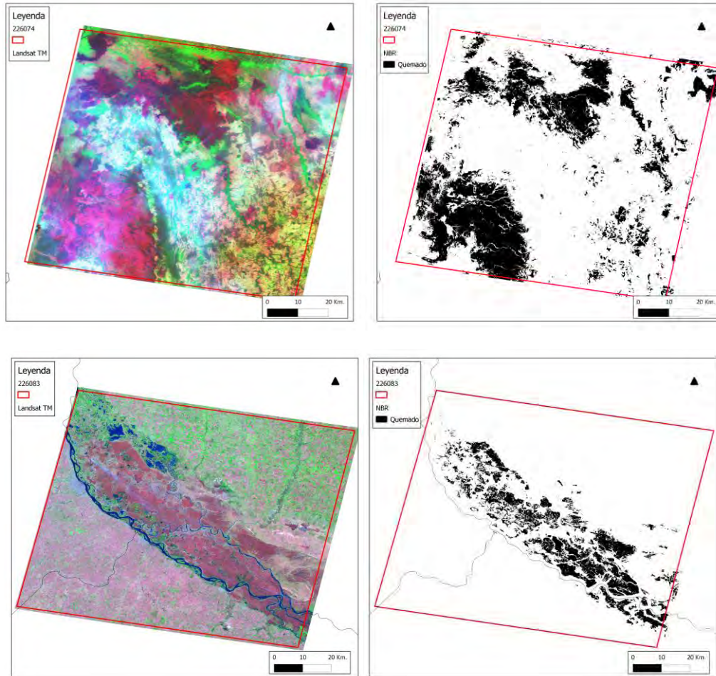
Figura 34: Arriba a la izquierda se presenta la composición en falso color de una imagen Landsat correspondiente al sitio de la ventana 226/074 en Brasil (RGB 7 4 3). A su derecha, el resultado de clasificar las áreas quemadas representadas en negro. Abajo la misma interpretación para el sitio correspondiente a la ventana 226/083 en el Delta del Paraná
