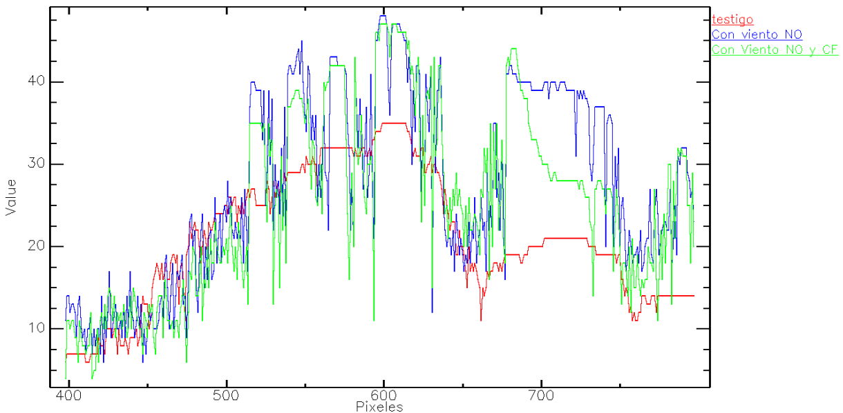
Figura 47: Perfiles longitudinales representativos de la frecuencia de píxeles quemados para tres modelos de índices de propagación. En rojo se presenta el caso testigo, en azul el caso con viento, y en verde el caso con viento y cortafuego.
