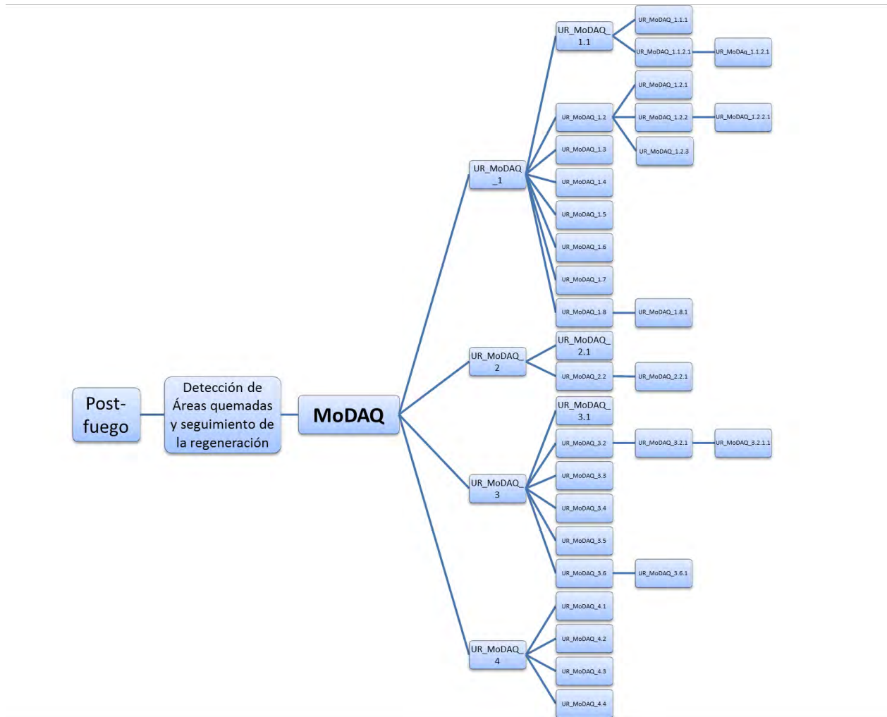
Figura 6: Esquema de la estructura sobre los requerimientos de usuarios correspondiente al módulo MoDAQ.
